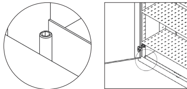
4 x Nivellierfüße von oben verstellbar mit einem Imbusschlüssel, Größe SW6
